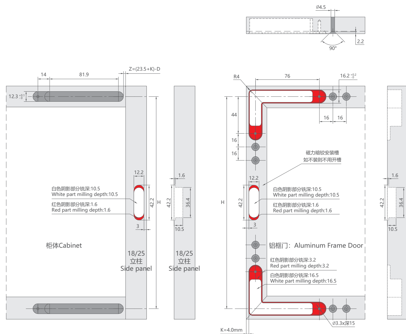
铝框门开孔尺寸 Dimensions of Aluminum frame door
