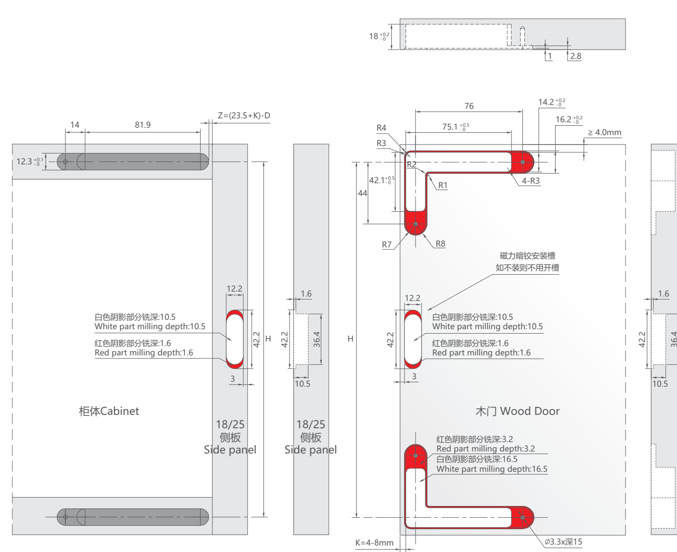
木门开孔尺寸 Dimensions of Wooden door
